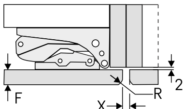
Fig. 69 Spárová štěrbina s navazujícími nábytkovými dvířky (F) Tloušťka čela (X) Spárová štěrbina min. (R) Rohový poloměr čela nábytku
