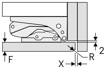
Fig. 68 Spárová štěrbina s navazujícím bočním dílem nábytku (F) Tloušťka čela (X) Spárová štěrbina min. (R) Rohový poloměr čela nábytku
