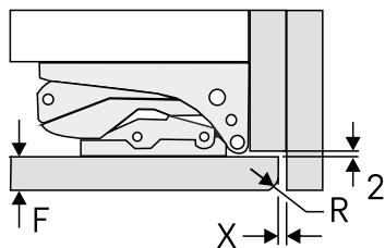
Fig. 66 Spárová štěrbina s navazujícím bočním dílem nábytku
