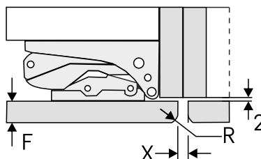
Fig. 67 Spárová štěrbina s navazujícími nábytkovými dvířky
