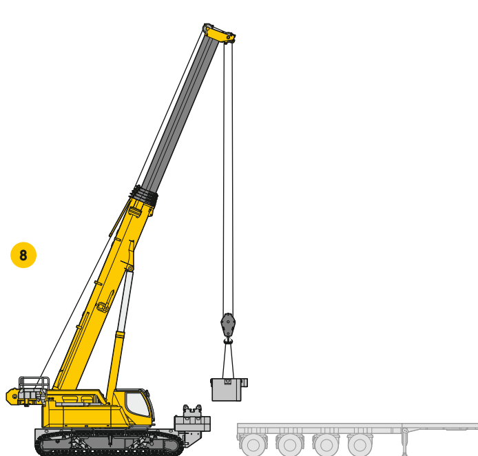
Montaje de la plataforma giratoria Монтаж балласта поворотной платформы
