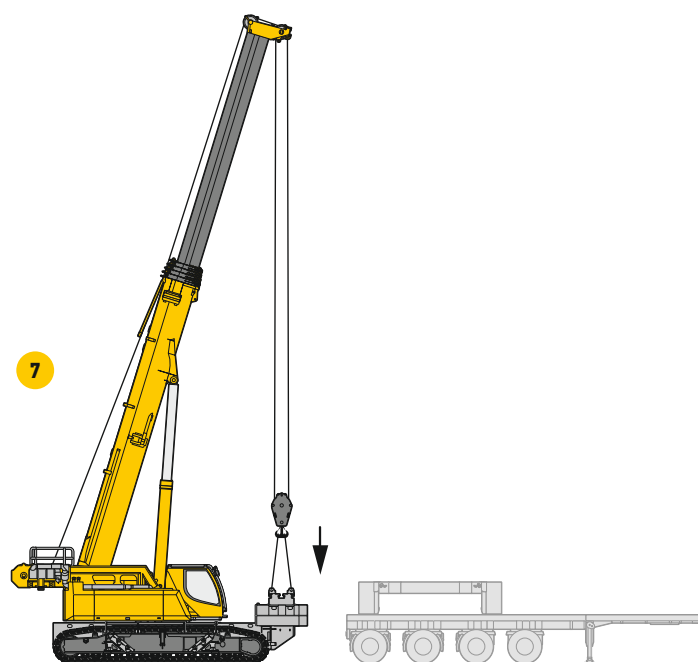
Montage Drehbühnenballast Assemble superstructure ballast
