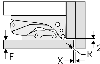
Fig. 67 Fugenspalt mit anschließender Möbelschwinge (F) Frontdicke (X) Fugenspalt min. (R) Eckradius Möbelschwinge
