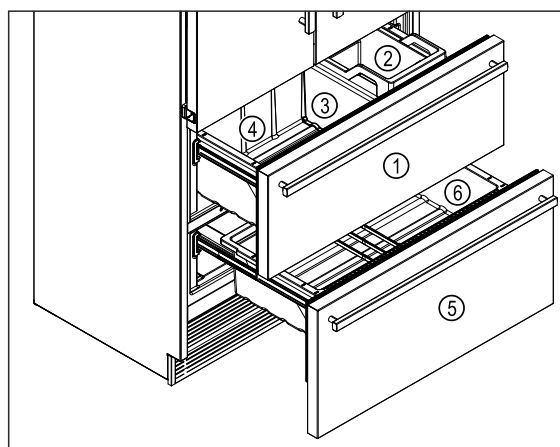
Fig. 63 Auszugswagen Gefrierteil
