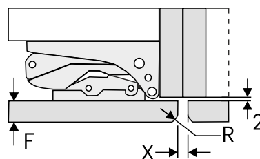
Fig. 66 Fugenspalt mit anschließender Möbeltür (F) Frontdicke (X) Fugenspalt min. (R) Eckradius Möbelfront
