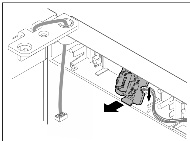
Fig. 18 Vous pouvez tourner le support de connecteur à 180° pour le monter dans la position inverse.*
