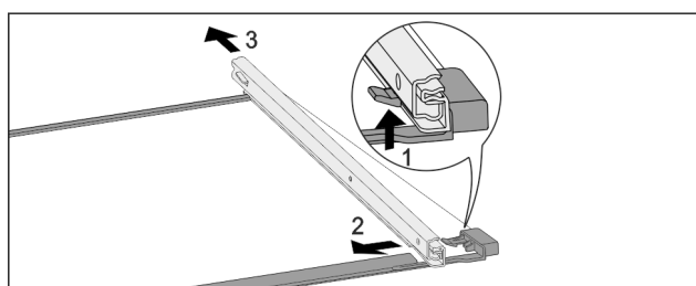
Fig. 230 Glasplatte mit Schienen
