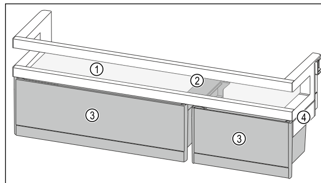
Fig. 180 Beispielhafte Darstellung Türabsteller mit VarioBoxen
