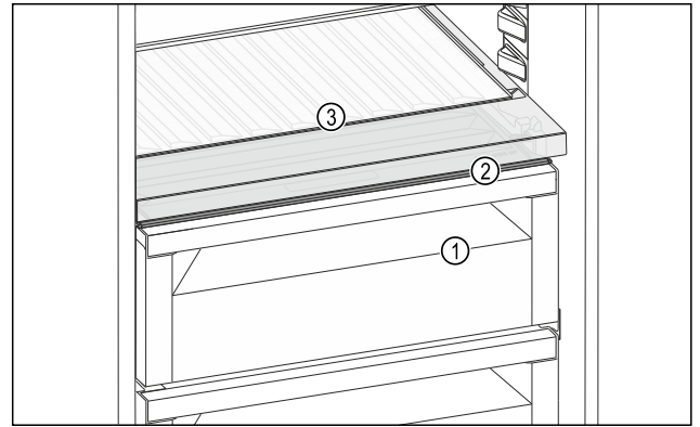
Fig. 204 Beispielhafte Darstellung Fachdeckel Fruit & Vegetable-Safe
