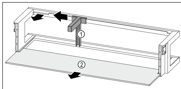
Fig. 226 Türabsteller mit Flaschenhalter und Abstellfläche
