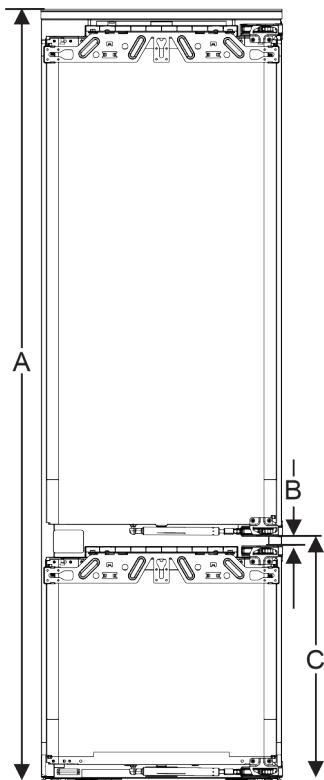
Fig. 65 Fugenlage zweitürige Möbeltür
