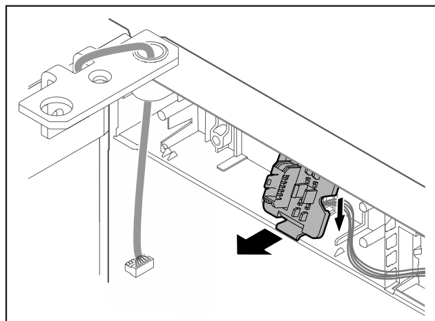
Fig. 20 La posizione di montaggio del supporto della spina può essere ruotata di 180°.*
