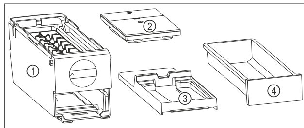
Sl. 173 Sastavni delovi EasyTwist-Ice aparata
