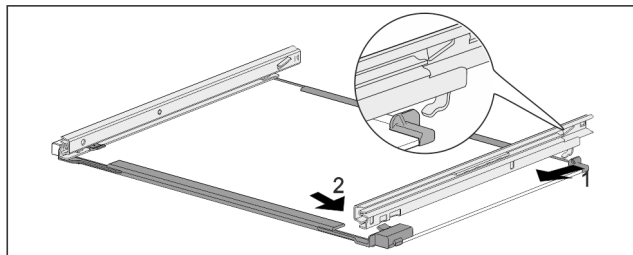
Sl. 236 Staklena ploča sa šinama
