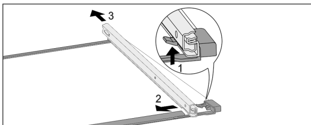
Sl. 235 Staklena ploča sa šinama
