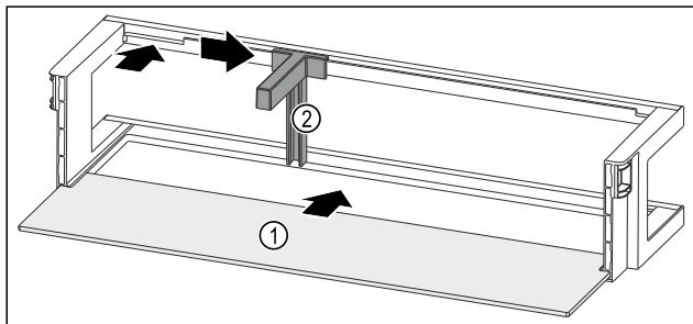
Sl. 234 Polica za vrata sa policom za odlaganje
