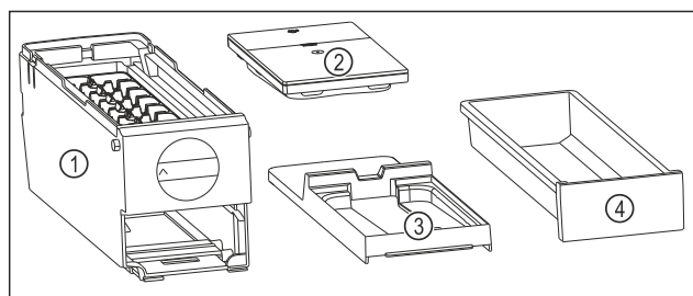
Sl. 244 Sastavni delovi EasyTwist-Ice aparata
