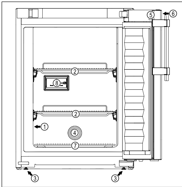
Fig. 1 Beispielhafte Darstellung: Gerät mit Auflageroste und Gerät mit Glasplatten und Schubfach
