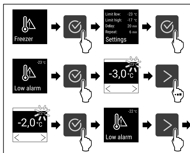
Fig. 129 Beispiel für die Einstellung der Temperaturuntergrenze, basierend auf einer eingestellten Gerätetemperatur von -20 °C.
