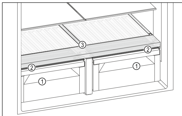
Fig. 127 Exemple illustré du couvercle du compartiment BioFresh
