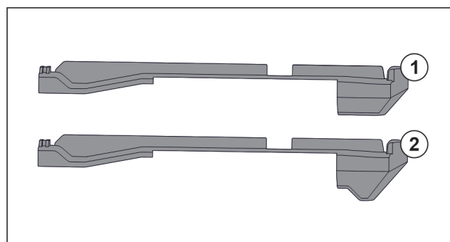
Fig. 83 Primerjava natičnih nastavkov
