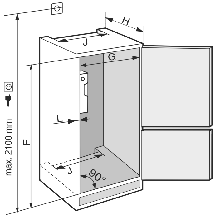
Фиг. 3
