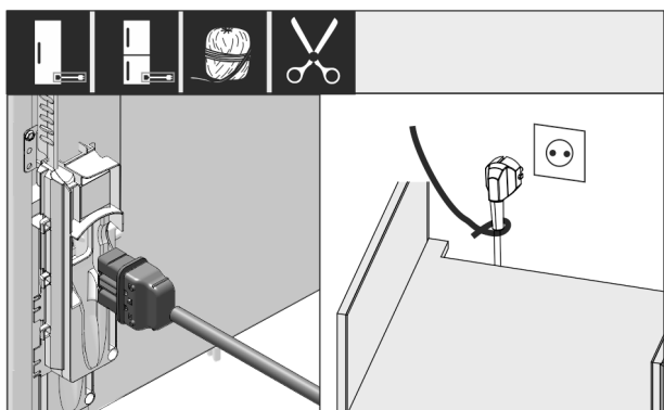
Фиг. 25
