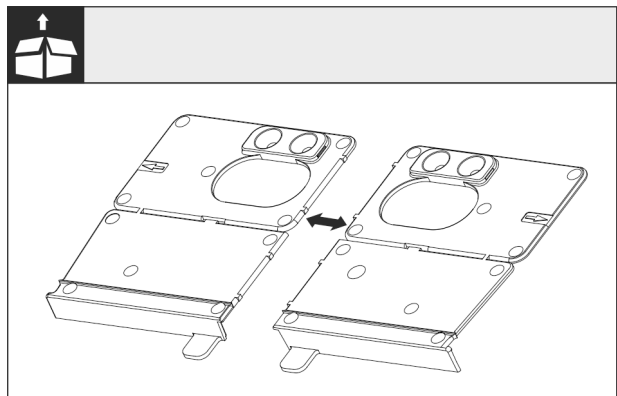
Фиг. 22 Монтажна винкла на подот
