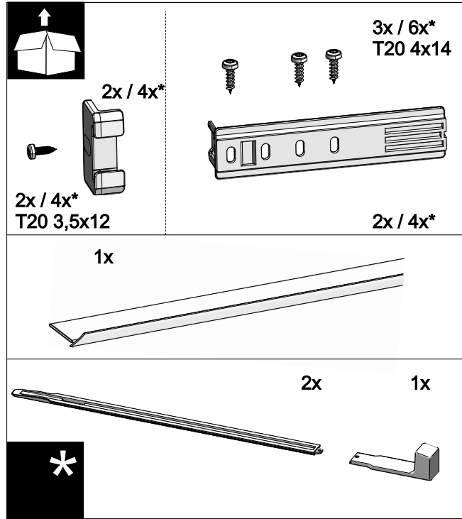
Фиг. 21
