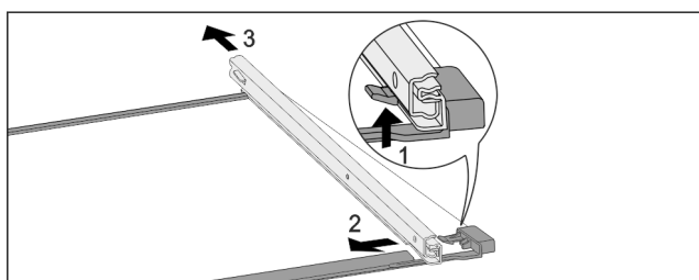
Fig. 122 Стъклена плоча със странични части
