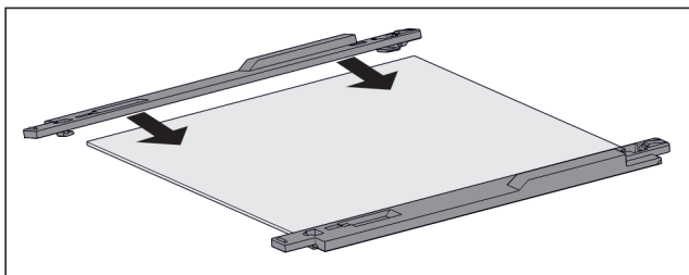
Fig. 130 Стъклена плоча със задържащи части
