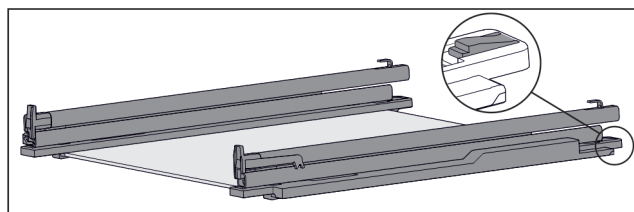
Fig. 64 Glasplatte mit Schienen und Halteteilen
