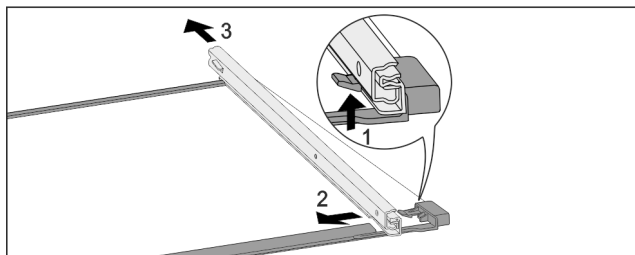
Fig. 55 Glasplatte mit Schienen
