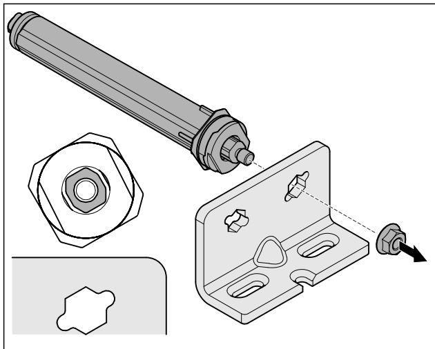
Fig. 23 Десен ограничител
