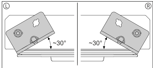
Fig. 41 Врата отдолу
