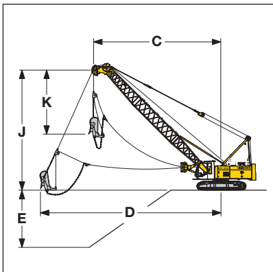
Traglasten in Tonnen (t) für Auslegerlängen von 11 m bis 26 m Ballast 12.8 t
