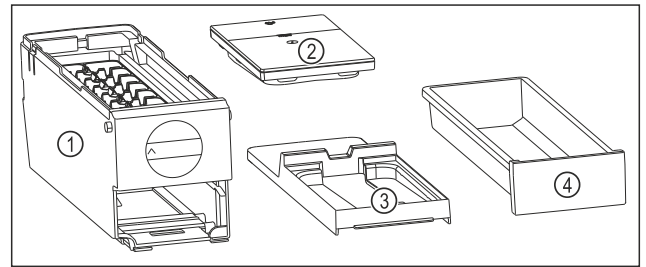
Fig. 89 EasyTwist-Ice'i koostisosad
