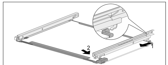
Fig. 83 Siinidega klaasplaat
