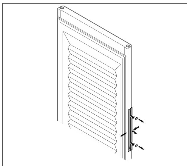
Fig. 13 Skumisoleret dør
