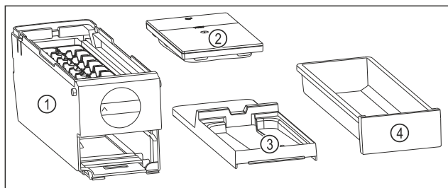
Fig. 185 Μέρη του EasyTwist-Ice
