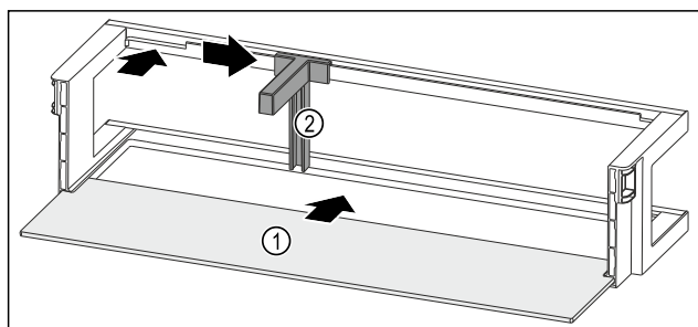
Fig. 89 Ράφι πόρτας με ράφι
