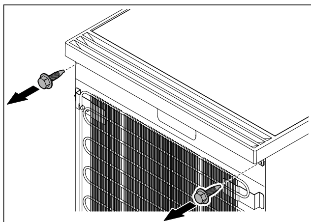
Fig. 15 ► 移除盖板 Fig. 15 (1)和 Fig. 15 (2)。
