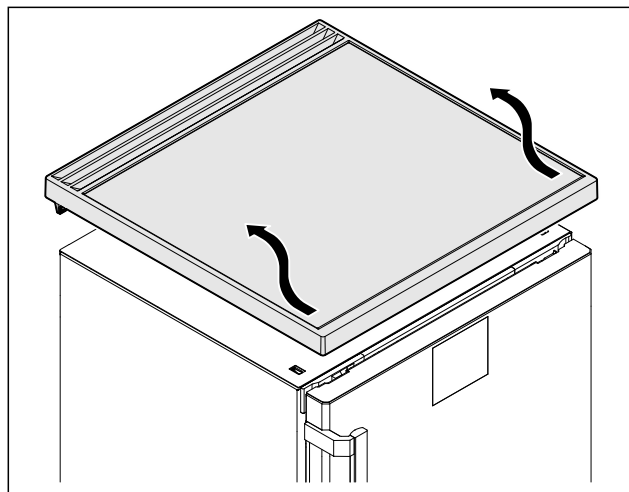
Fig. 13 ► 移除工作台面。
