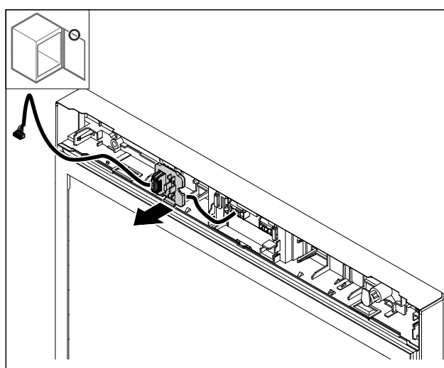
Fig. 28 Stikholderens monteringsposition kan være drejet 180°.
