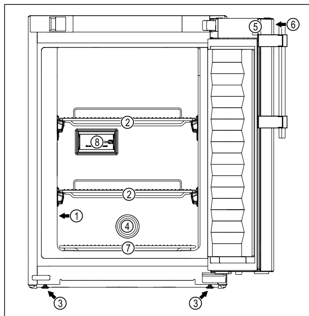
Fig. 1 Vejledende illustration: Enhed med rist og enhed med glasplader og skuffe
