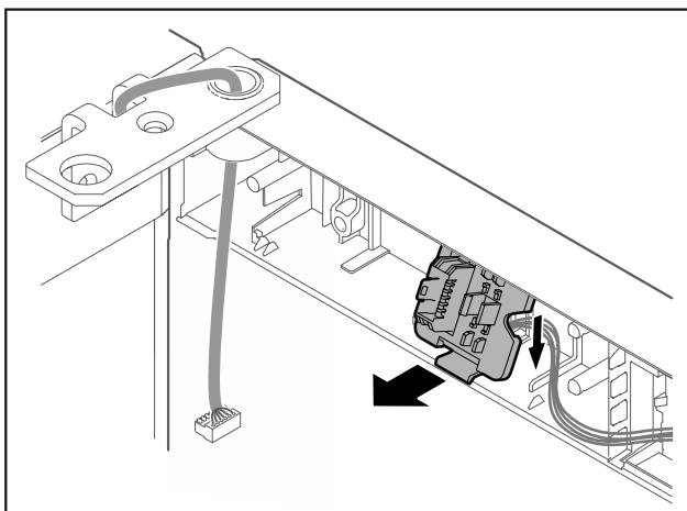
Fig. 23 Kištuko laikiklio montavimo padėtį galima pasukti 180°.
