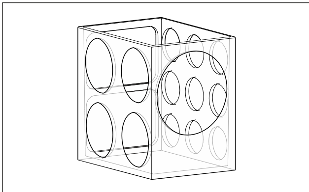
Fig. 66 Voorbeeldweergave
