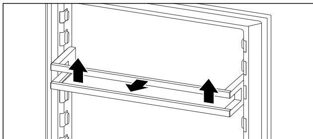
Fig. 51 Voorbeeldweergave
