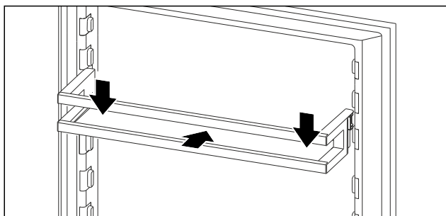
Fig. 52 Voorbeeldweergave
