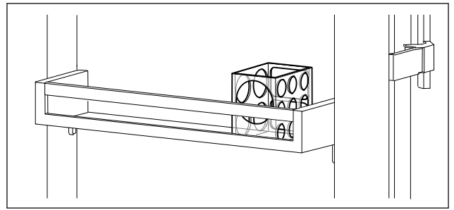
Fig. 67 Voorbeeldweergave
