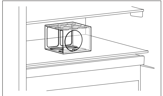
Fig. 68 Voorbeeldweergave
