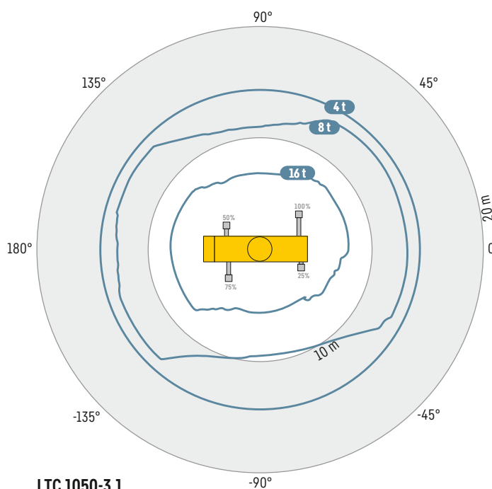
LTC 1050-3.1
