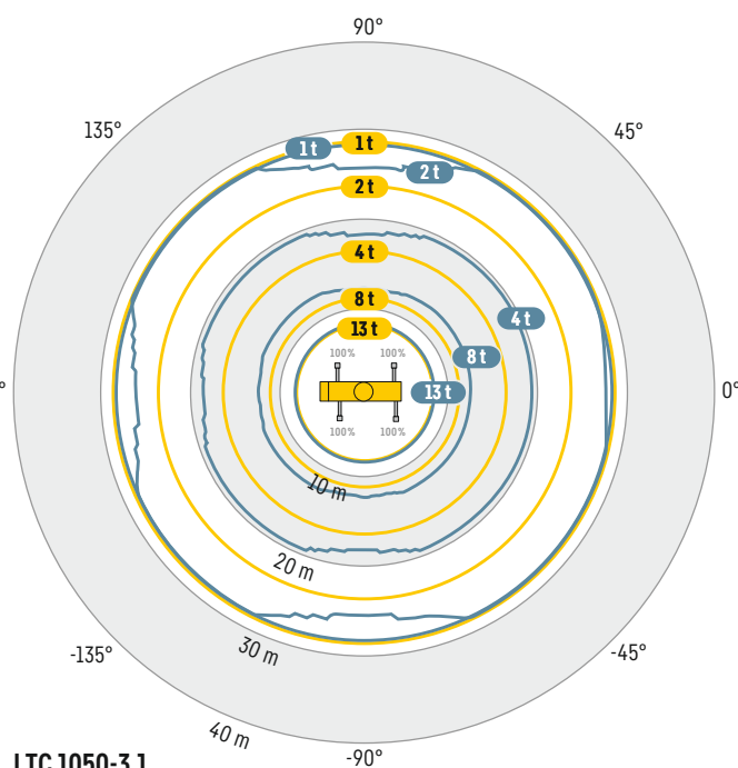
LTC 1050-3.1
