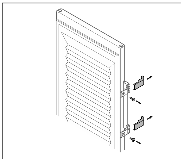
Fig. 27 Geschäumte Tür
