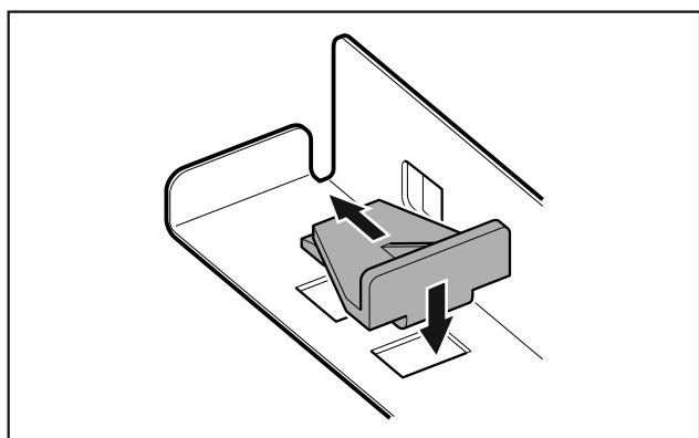
Fig. 57 Anschlagwinkel einsetzen
