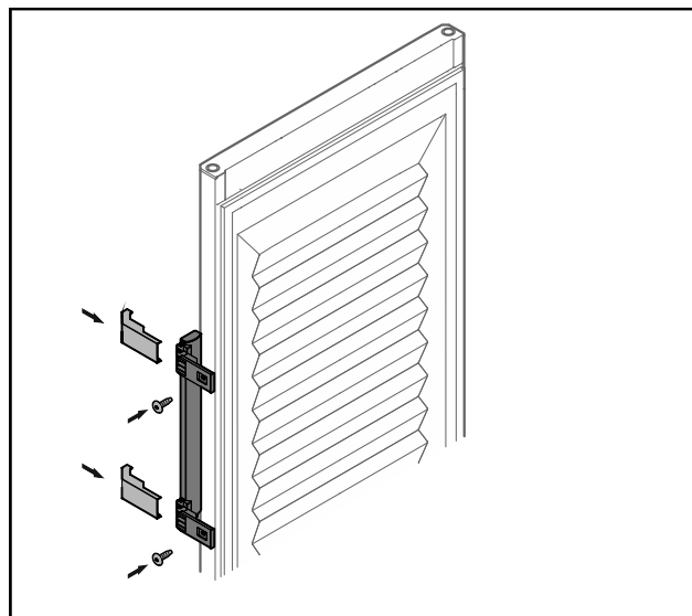
Fig. 29 Geschäumte Tür
