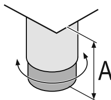
Fig. 12 De stelvoet is van A = 115 mm (4 1/2 in) tot 175 mm (6 7/8 in) verstelbaar.
