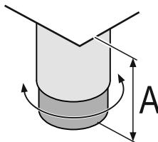
Fig. 10 Seřizovací nožku lze přestavět od A = 115 \text{ mm} ( 4 \frac{1}{2} \text{ in} ) do 175 \text{ mm} ( 6 \frac{7}{8} \text{ in} ).
