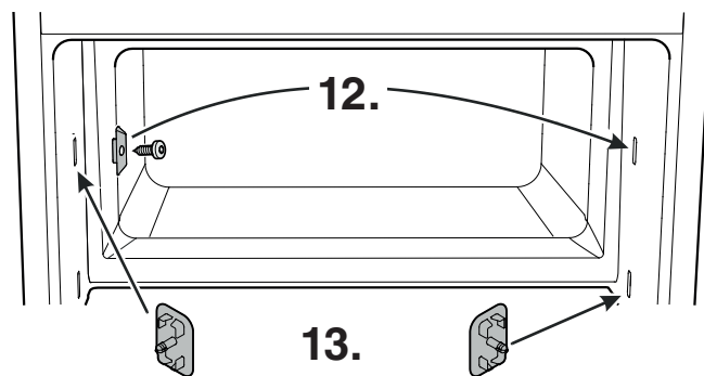
12. Spostare il gancio di chiusura.
