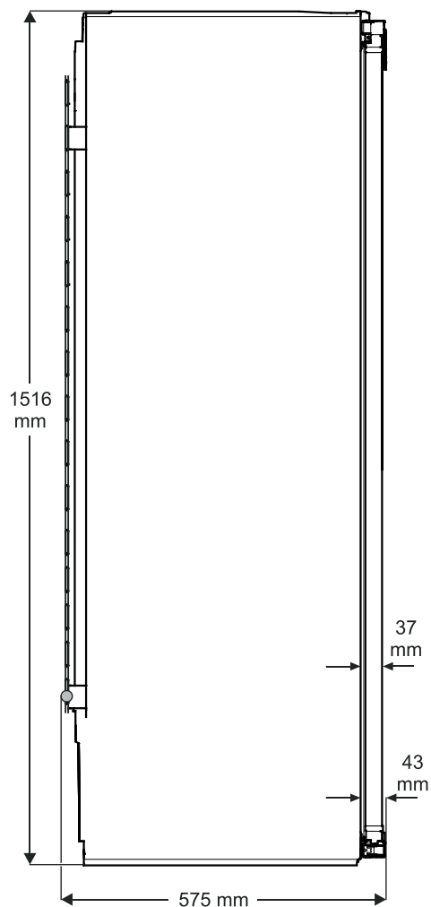
Vista laterale
