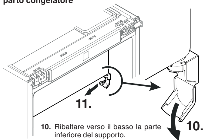
11. Allentare la vite.
