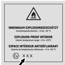
Fig. 3 防护等级: II 3/-G Ex ec IIC T6 Gc/-
