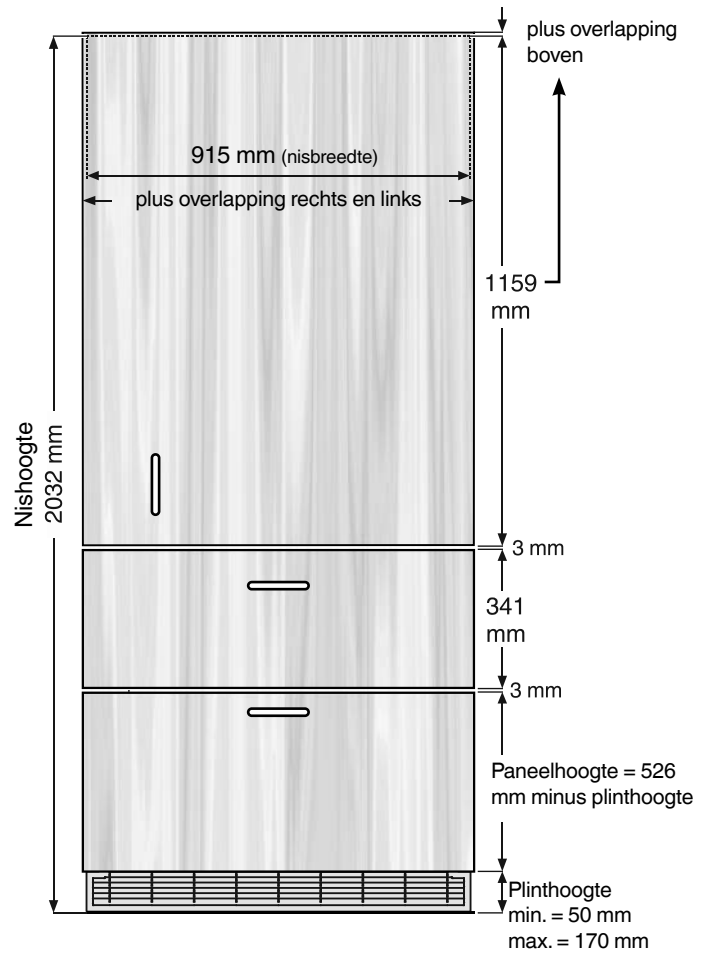
Buitenliggend deurpaneel
