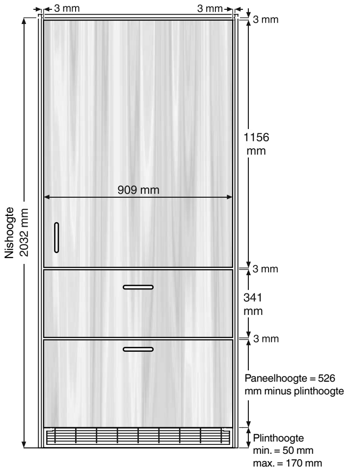
Binnenliggend deurpaneel
