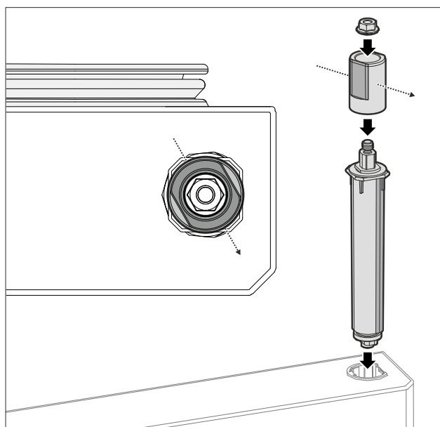
Fig. 57 Høyre anslag
