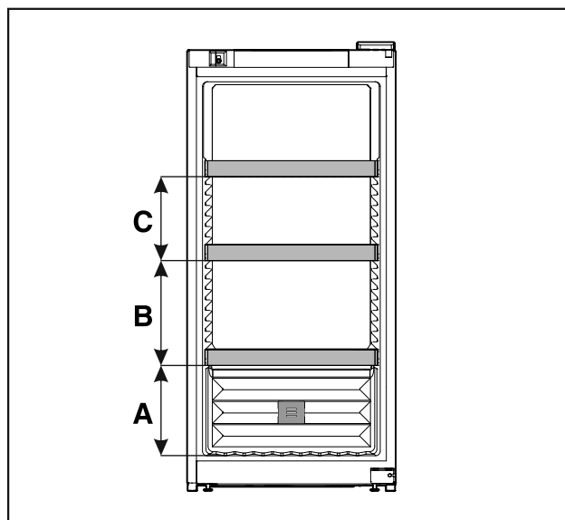
Fig. 6 Razmiki med pokrivnimi rešetkami
