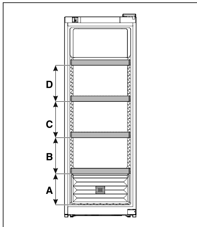
Fig. 12 Razmiki med pokrivnimi reškami
