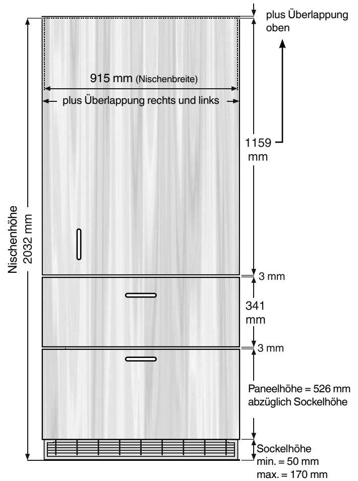
Außenliegendes Türpaneel
