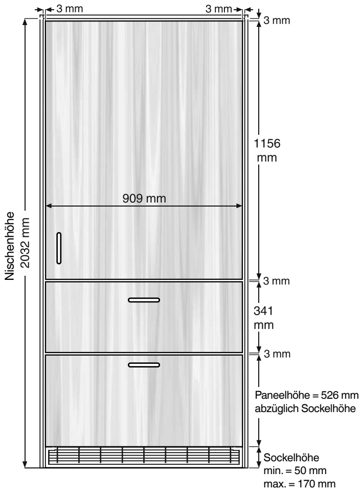
Innenliegendes Türpaneel
