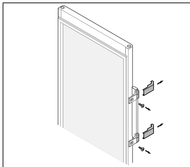
Fig. 27 Zapěnění dvířka*
