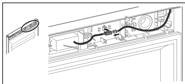
Fig. 38 Ușă spumată
