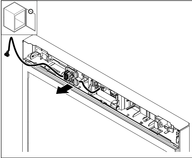
Fig. 29 插头架的安装位置可以转动180°。
