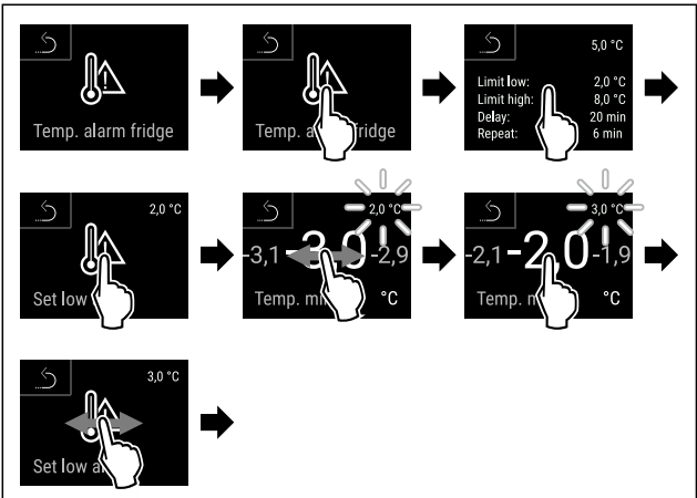
Fig. 178 设置温度下限的示例，基于 5 °C 的已设置的冰箱温度。
