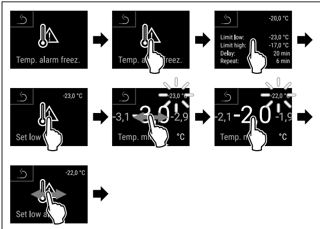
Fig. 185 设置温度下限的示例，基于 -20 °C 的已设置的冰箱温度。
