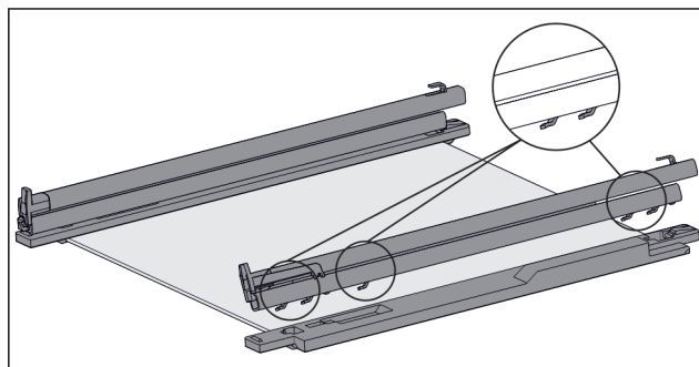
Fig. 150 Skleněná deska s kolejnicemi a přídržnými díly
