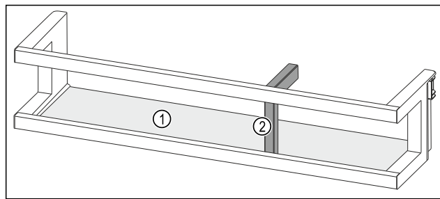
Fig. 77 Ενδεικτική απεικόνιση ραφιού πόρτας με στήριγμα φιαλών
