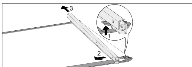
Fig. 125 Γυάλινο ράφι με ράγες
