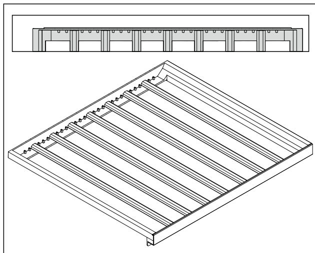
Fig. 90 Uspořádání lišt pro maximální počet lahví.
