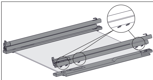
Fig. 150 Sklenená doska s koľajničkami a prídržnými dielmi
