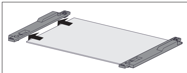
Fig. 117 Glasplatte mit Schienen und Halteteilen
