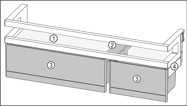
Fig. 84 带 VarioBox 的门边存放架例图 (1) 搁板 (3) VarioBox (2) VarioBox 定位件 (4) 侧面部分
