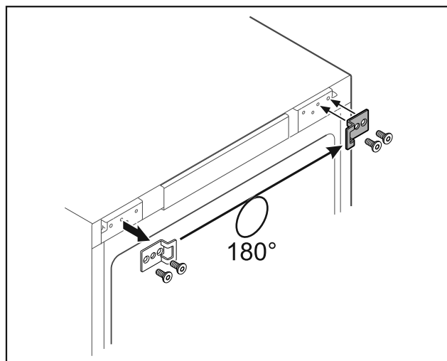
Fig. 31 Puerta con plástico espumado
