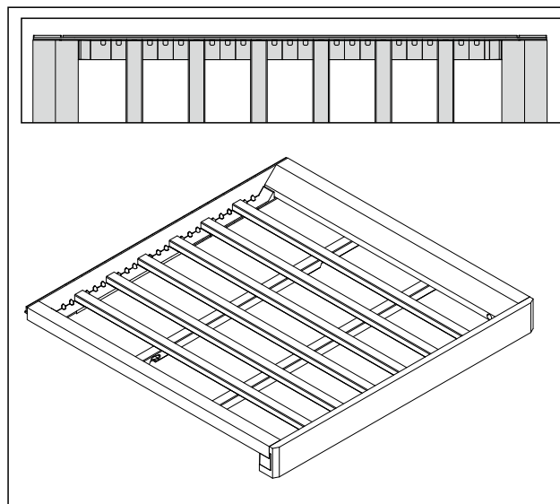
Fig. 94 Uspořádání lišt pro maximální počet lahví.
