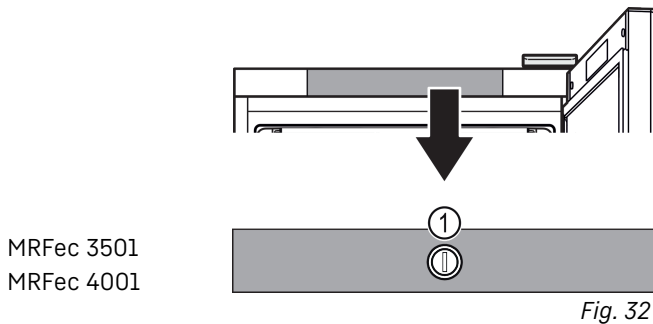
Fig. 32 (1) Ρυθμιστής θερμοκρασίας
